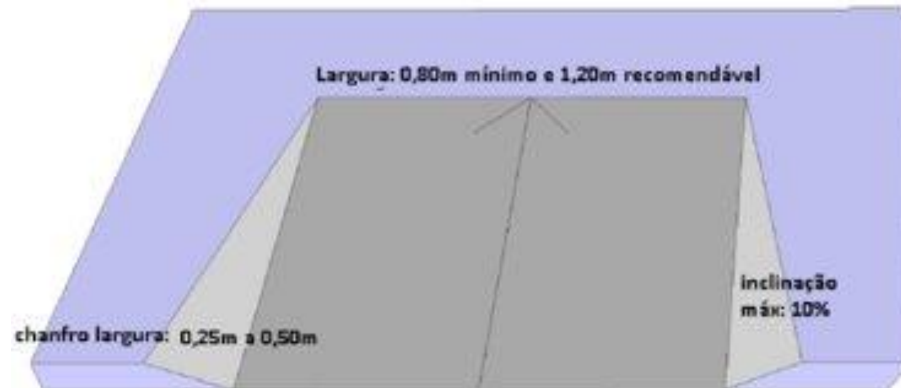
Rampa com acabamento chanfrado
